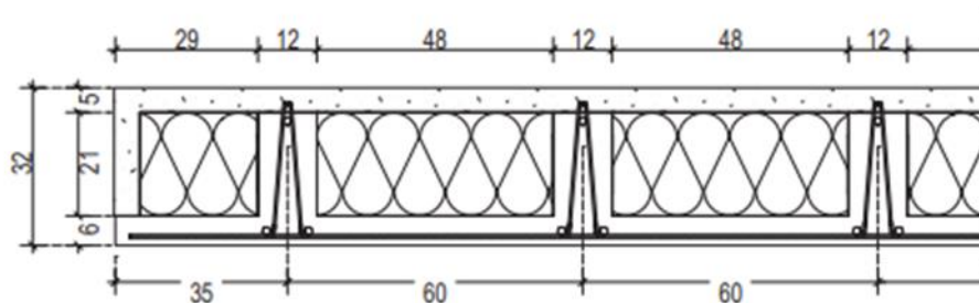
Figure : Coupe du plancher dalle BB complet. Epaisseur Dalle BB : 27 cm.
